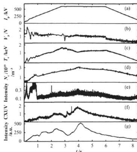
图 7 欧姆放电 #36409 炮放电波形 (a) 等离子体电流, (b) 环电压, (c) 电子温度, (d) 中心弦平均电子密度, (e) C III(4 647 Å) 线辐射强度, (f) XUV 辐射强度, (g) C IV(312.42 Å) 线强度随时间演化 Fig.7 Waveforms of shot 36409# discharge. (a) Plasma current, (b) Cycle voltage, (c) Electron temperature, (d) Average density of electron along centre chord, (e) Time evolution of C III (4 647 Å), (f) Time evolution of XUV radiation intensity, (g) Time evolution of C IV (312.42 Å)
