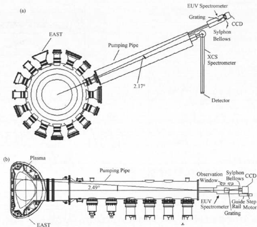
图 4 EUV 在 EAST 安装示意图(俯视图)(a)和(侧视图)(b) Fig.4 EUV spectrometer on EAST (top view) (a) and (side view) (b).
