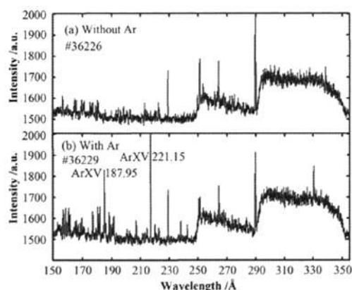
图 6 EAST 装置放电期间采到的原始谱线 Fig.6 EUV spectra from EAST discharges.
